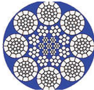
Figura 3: Corte transversal 8x37 FS (exterior plastificado)
