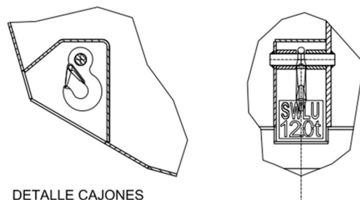
DETALLE CAJONES GANCHO ELEVACIÓN.
